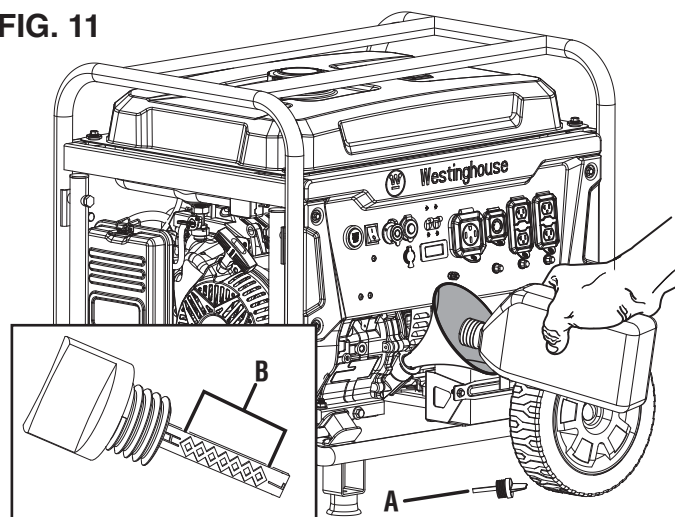
A - Jauge d'huile B - Plage de fonctionnement sûre
