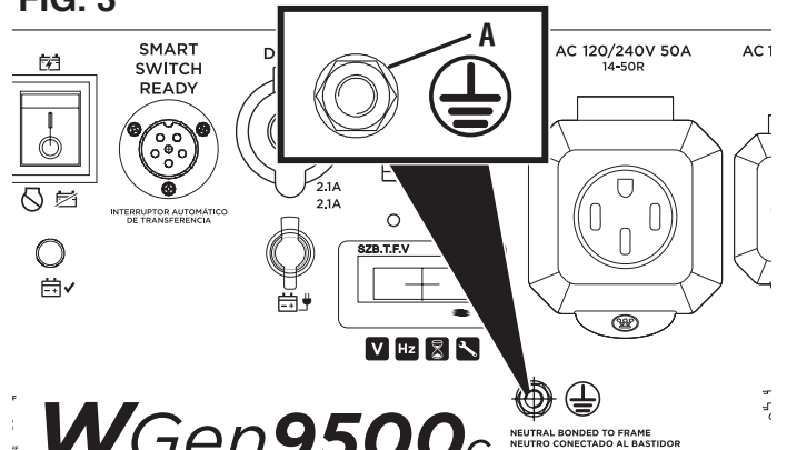
A - Borne mise à la terre
