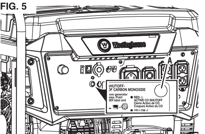
A - VOYANT LUMINEUX DU CAPTEUR DE CO
