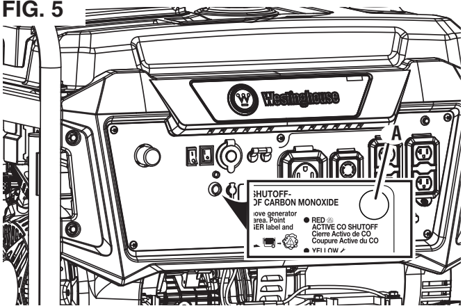
A - INDICATEUR LUMINEUX DU CAPTEUR DE CO
