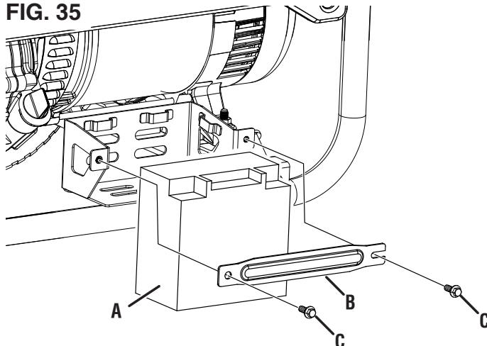
A - Batterie B - Plaque de batterie C - Boulon
