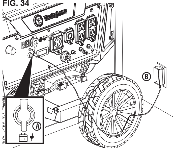
A - Port de chargement de la batterie B - Chargeur
