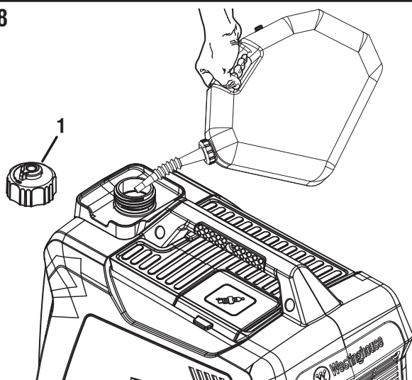
1 - Bouchon de réservoir ventilé
