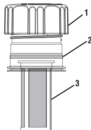
1 - Bouchon de réservoir ventilé 2 - Ligne de remplissage maximale 3 - Filtre d'écran
